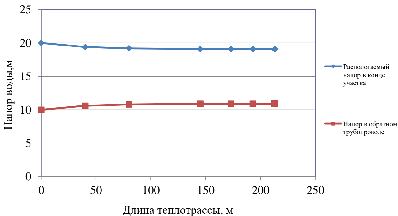
Рисунок 2.6 – Пьезометрический график тепловой сети котельной с. Усть-Каменка
