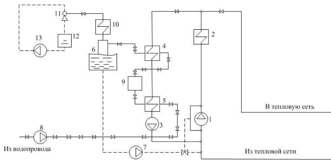
1 - сетевой насос; 2 - водогрейный котел; 3 - рециркуляционный насос; 4 - подогреватель подпиточной воды; 5 - подогреватель водопроводной воды; 6 - вакуумный деаэратор; 7 - подпиточный насос и регулятор подпитки; 8 - насос водопроводной воды; 9 - оборудование химводоподготовки; 10 - охладитель выпара; 11 - вакуумный водоструйный эжектор; 12 – бак газоотделитель эжектора; 13 - эжекторный насос
