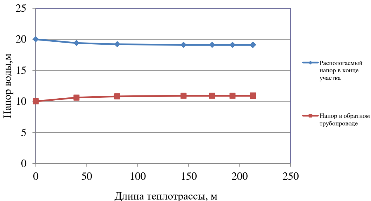
Рисунок 2.5 – Пьезометрический график тепловой сети котельной с. Усть-Каменка
