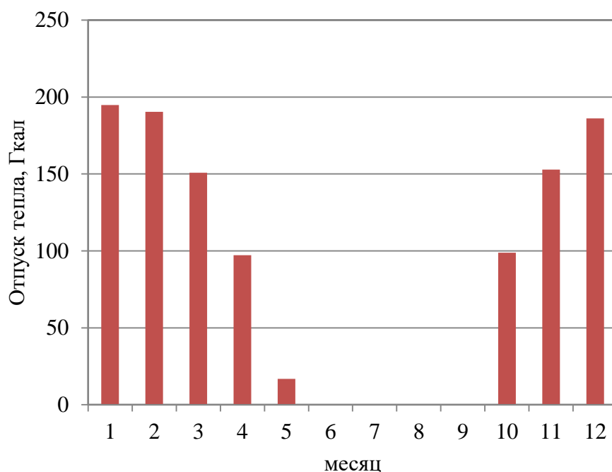
Рисунок 1.3 – Оптимальный температурный график системы теплоснабжения для котельной с. Усть-Каменка
