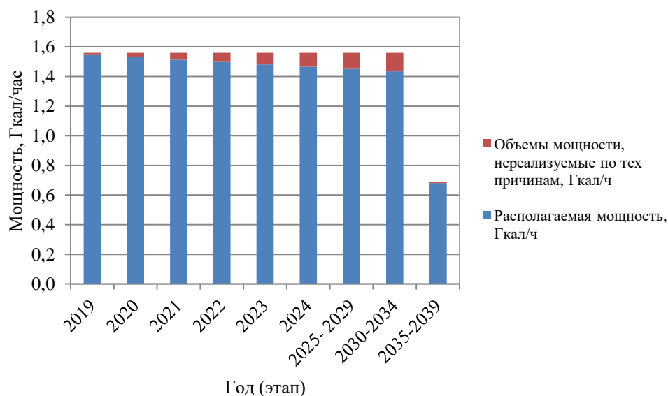
Рисунок 1.2 – Перспективные балансы тепловой мощности источников тепловой мощности и тепловой нагрузки потребителей котельной с. Усть-Каменка
